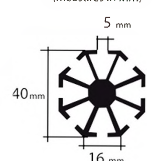
PERFIL VERTICAL VERTICAL PROFILE (medidas en mm) (measures in mm)
