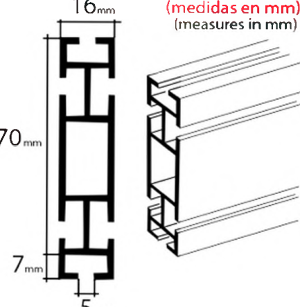
BANDA HORIZONTAL HORIZONTAL BAND (medidas en mm) (measures in mm)
